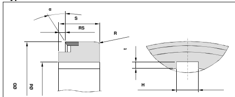
Typ NN-HM mit Nut
