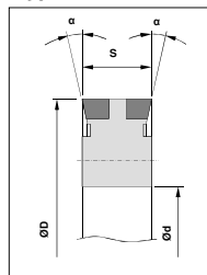
Typ UN-HM
