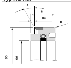
Typ NG-HM
