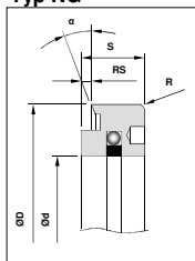
Typ NG
