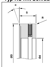
Typ NS mit Schraubfeststellun Typ NS-HM mit Schraubfeststellung
