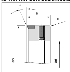
Typ NS mit Schraubfeststellun Typ NS-HM mit Schraubfeststellung
