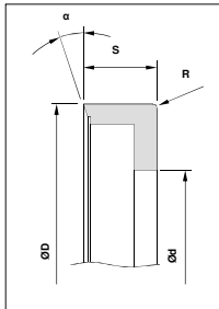
Topfmesser
