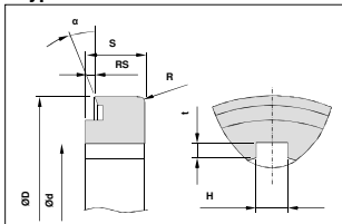
Typ NN mit Nut
