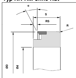
Typ NN-HM ohne Nut
