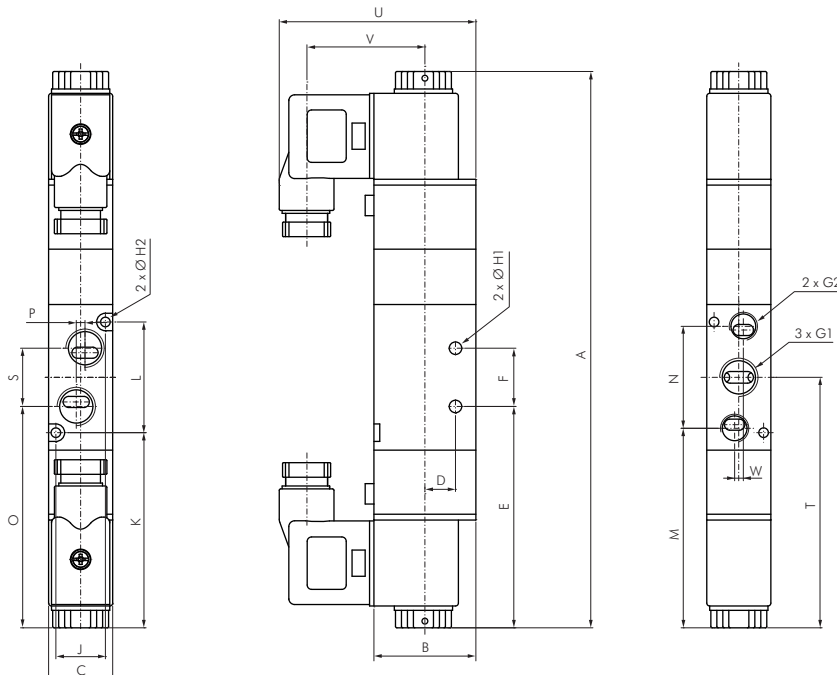
5/3-Wege Ventil
