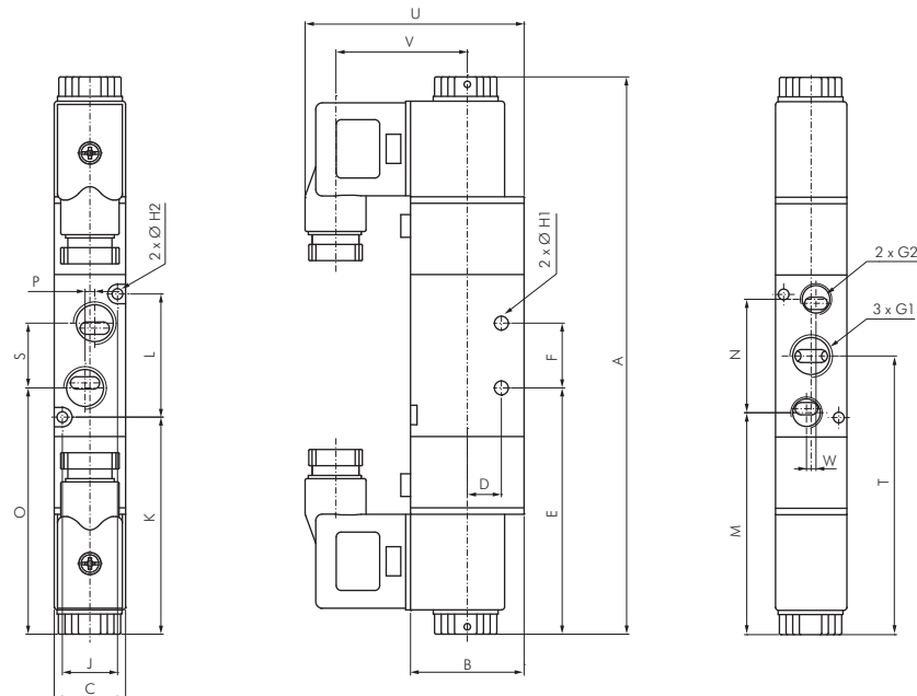
5/2-Wege Impulsventil
