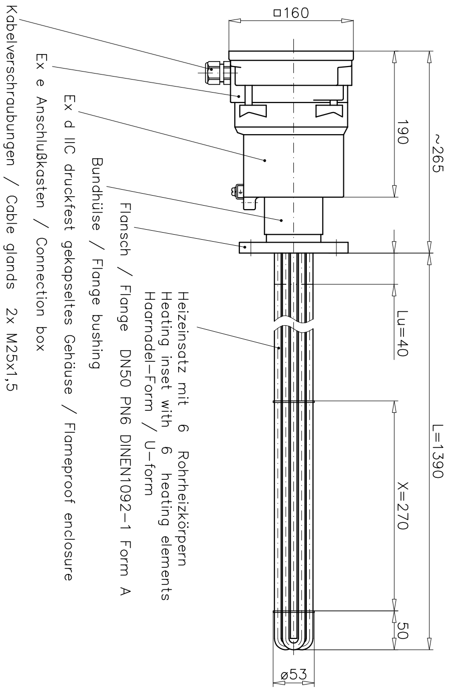
Elektrischer Anschlussraum Electrical connection box
