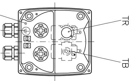
Ansicht ohne Anschlusskastendeckel View without connection box cover
